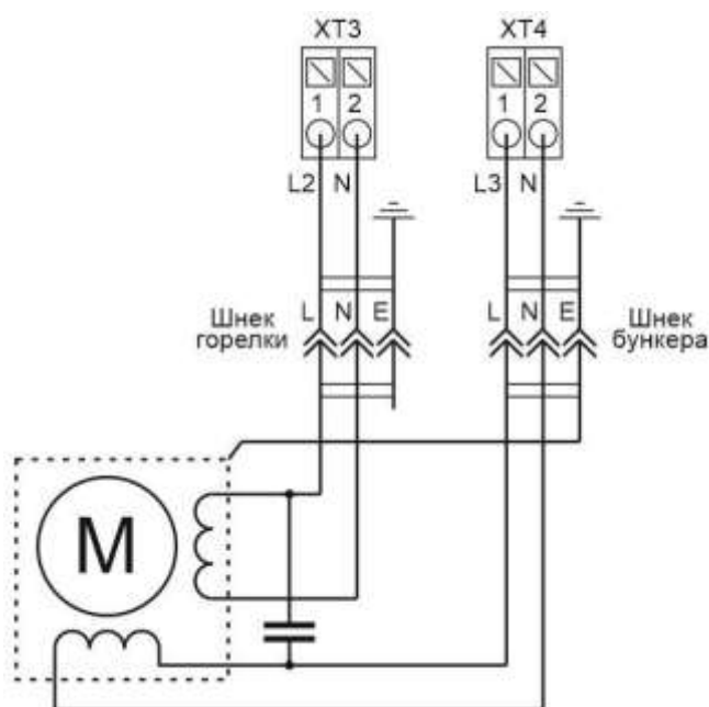
Подключение шнеков при использовании функции «Антиблок»
