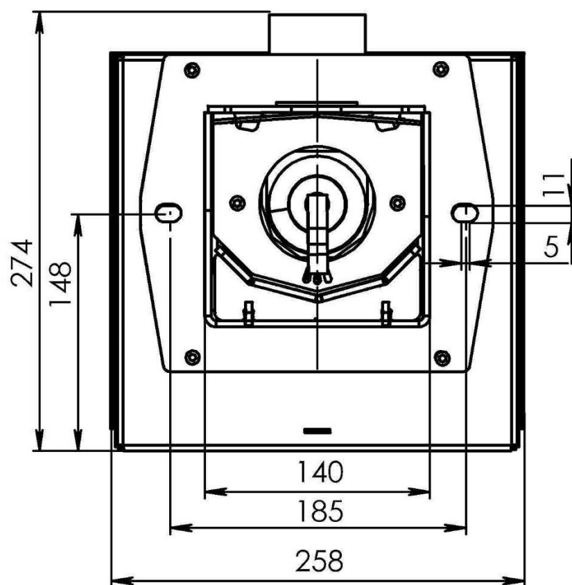
Рисунок 2 - Габаритные размеры горелки
