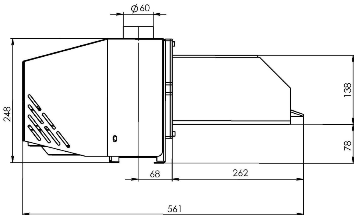
Рисунок 2 - Габаритные размеры горелки
